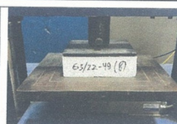
Рисунок 3 – Загальний вигляд зразків № 63/22 під час випробування
