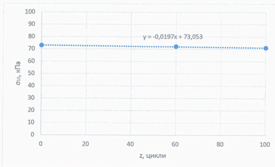
Рисунок 6 – Залежність міцності на стиск при 10% деформації від циклічних впливів для зразків будівельного теплоізоляційного матеріалу марки EPS 70 (TM Eurobud, TM Styrotherm, TM Ecotherm, TM BauGut) виробництва ПП «ЗАВОД «ПІНОПЛАСТ»
