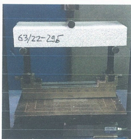
Рисунок 7 – Проведення випробування та типова експериментальна залежність при визначенні міцності при згині зразків теплоізоляційного матеріалу марки EPS 70 (TM Eurobud, TM Styrotherm, TM Ecotherm, TM BauGut) виробництва ПП «ЗАВОД «ПІНОПЛАСТ»
