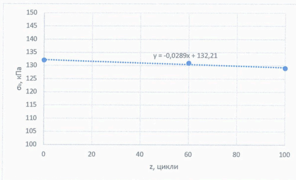
Рисунок 8 – Залежність міцності при згині від циклічних впливів для зразків будівельного теплоізоляційного матеріалу марки EPS 70 (TM Eurobud, TM Styrotherm, TM Ecotherm, TM BauGut) виробництва ПП «ЗАВОД «ПІНОПЛАСТ»
