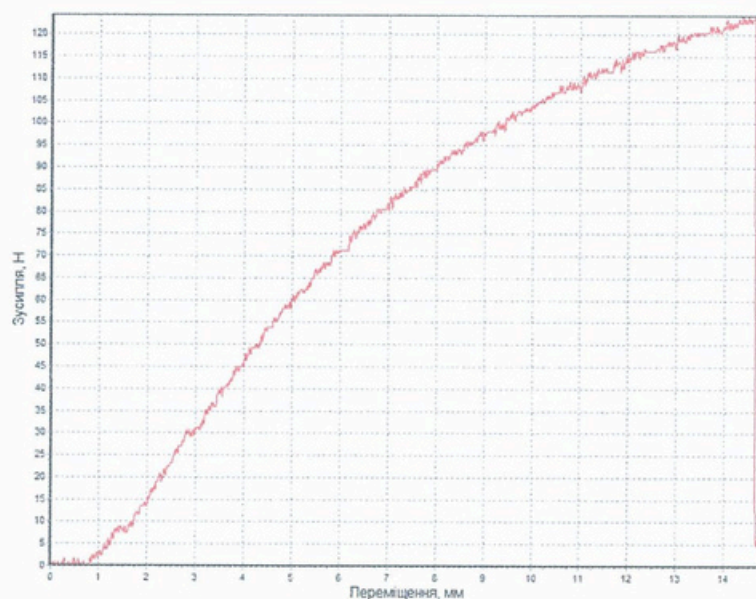
Рисунок 7 – Проведення випробування та типова експериментальна залежність при визначенні міцності при згині зразків теплоізоляційного матеріалу марки EPS 70 (TM Eurobud, TM Styrotherm, TM Ecotherm, TM BauGut) виробництва ПП «ЗАВОД «ПІНОПЛАСТ»
